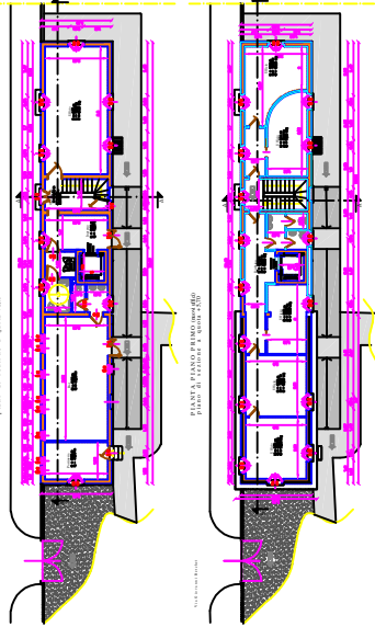
PIANO DI FASCIA DI CALZATA PIANO DI FASCIA DI CALZATA PIANO DI FASCIA DI CALZATA
