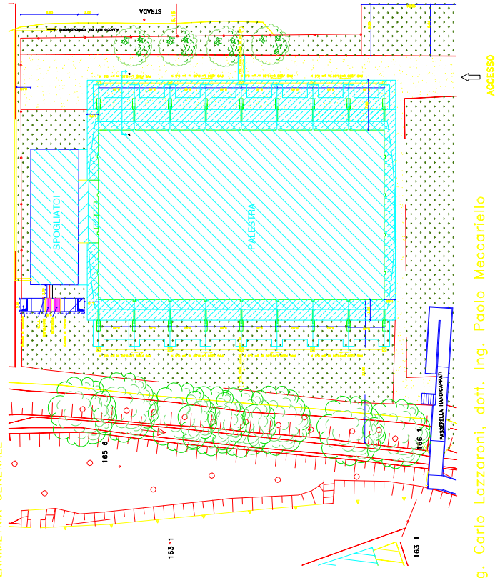
PLANIMETRIA GENERALE
