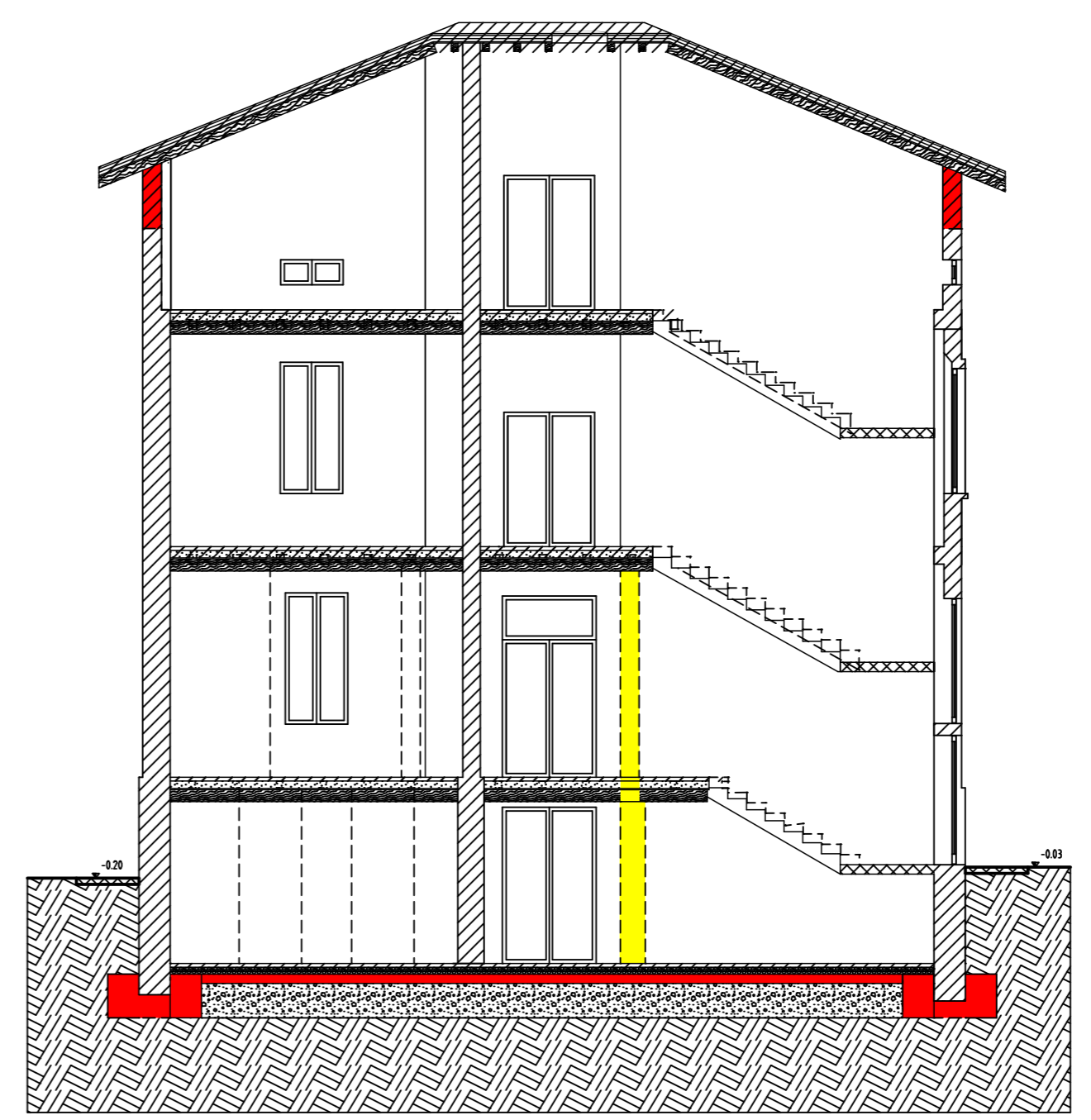
SEZIONE A-A SOVRAPPOSIZIONE
