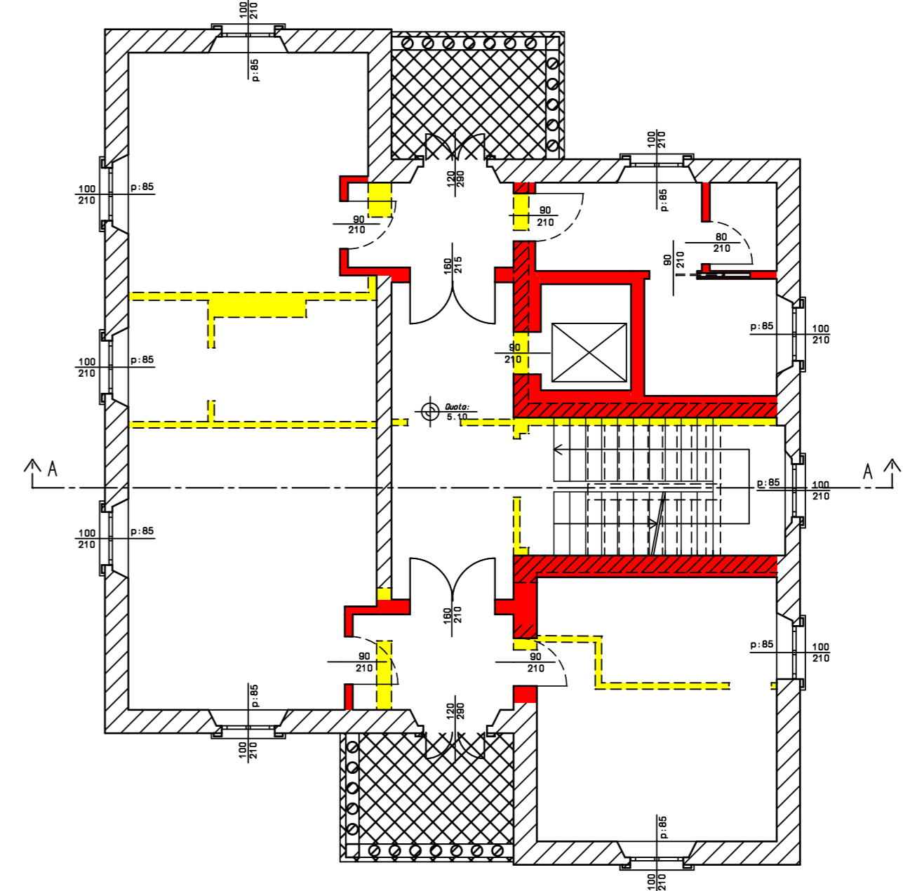
PIANO PRIMO: SOVRAPPOSIZIONI
