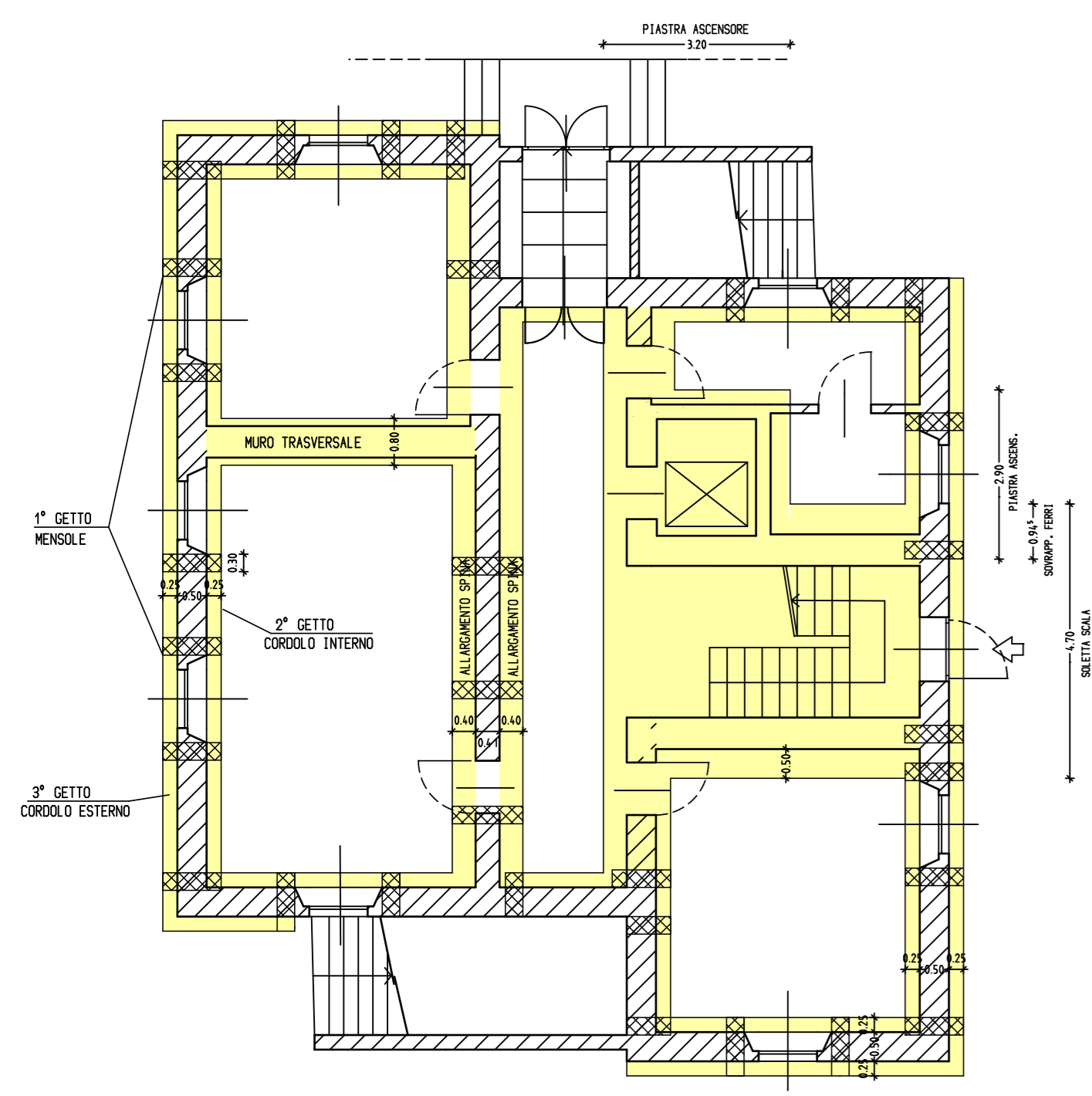
PIANO SEMINTERRATO: SOTTOMURAZIONI
