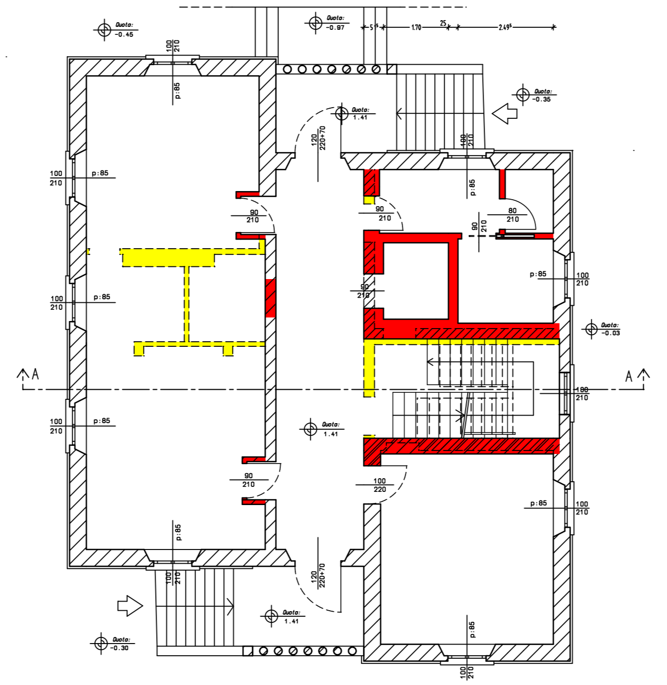
PIANO RIALZATO: SOVRAPPOSIZIONI
