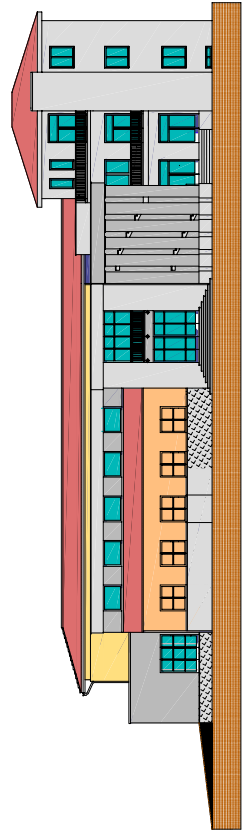
PROSPETTO EST
